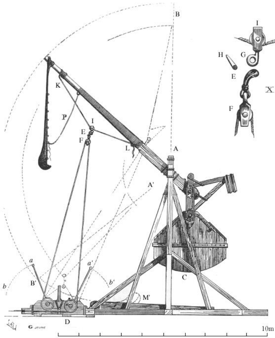
回回砲(Trebuchet)
